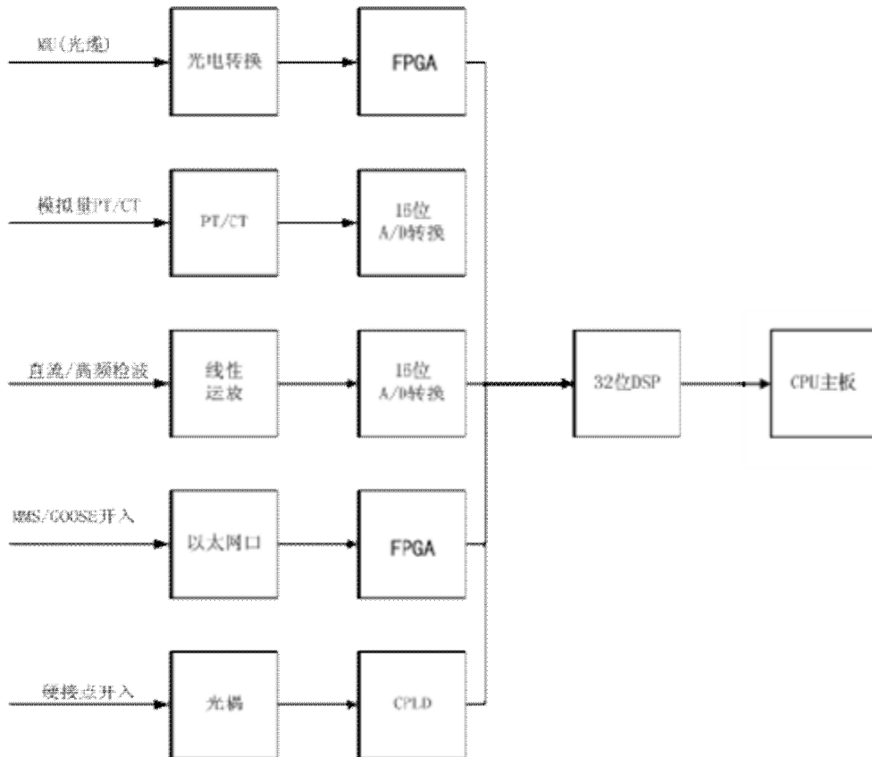
图 2.1-1 信号输入
